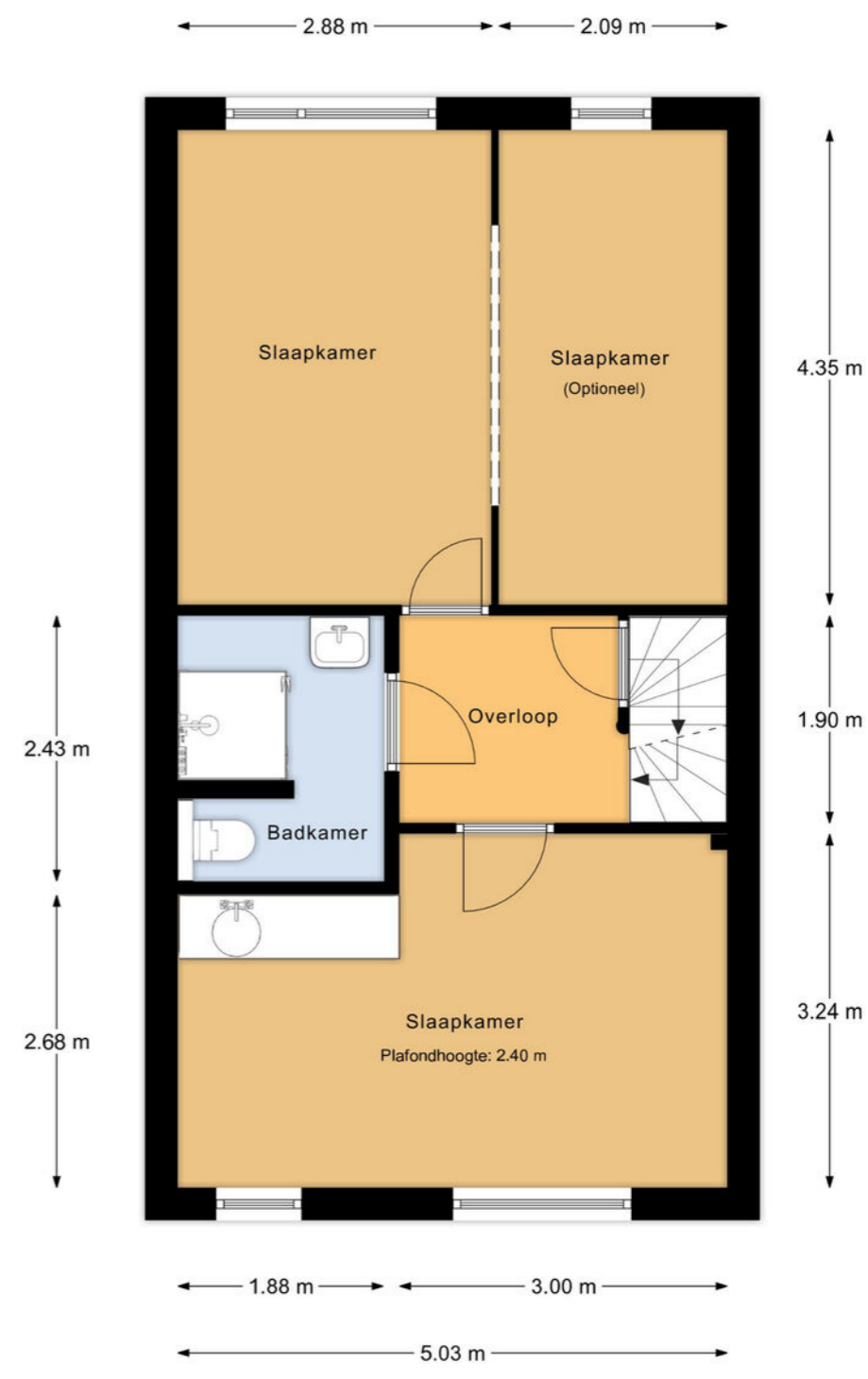
1e Verdieping
