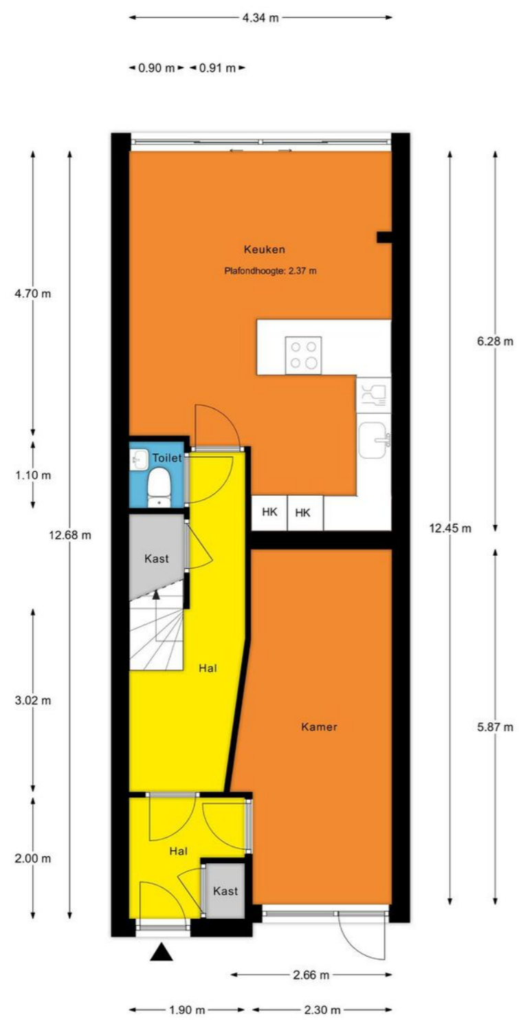
Begane Grond MAATVOERINGEN ZIJN INDICATIEF Aan deze tekening kunnen geen rechten worden ontleend
