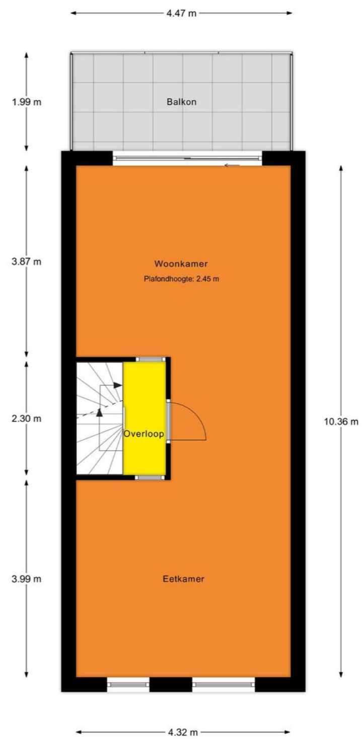
1e Verdieping MAATVOERINGEN ZIJN INDICATIEF Aan deze tekening kunnen geen rechten worden ontleend
