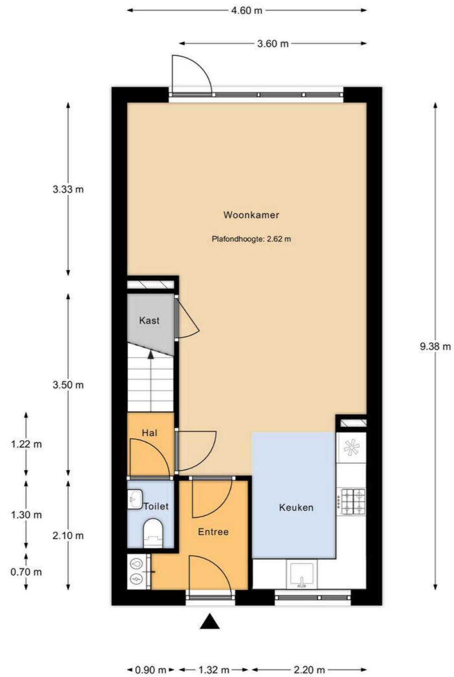
Begane Grond
