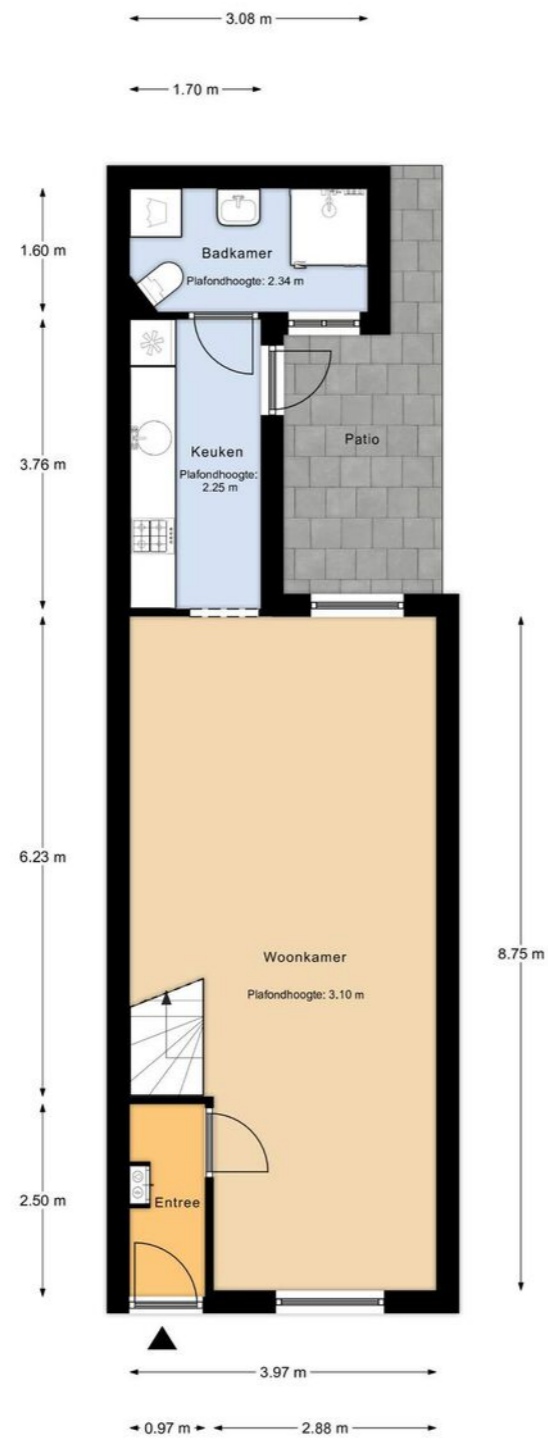
Perceeloverzicht
